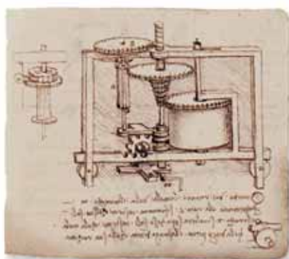
Леонардо да Винчи. “Механизмы”. Технический рисунок
